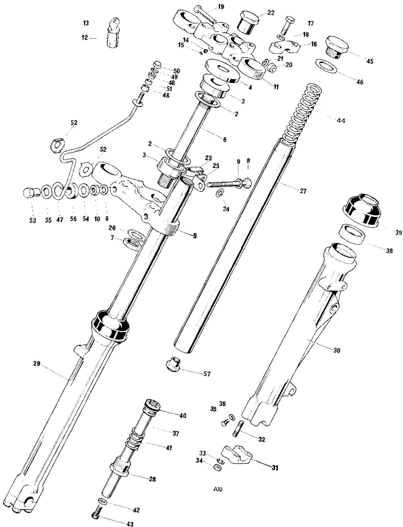
Fig. 10. TELESCOPIC FORKS
