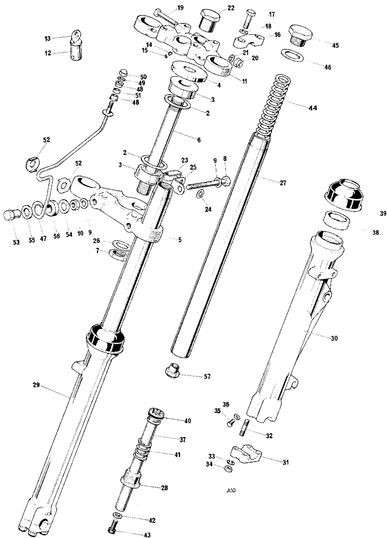
Fig. 10. TELESCOPIC FORKS
