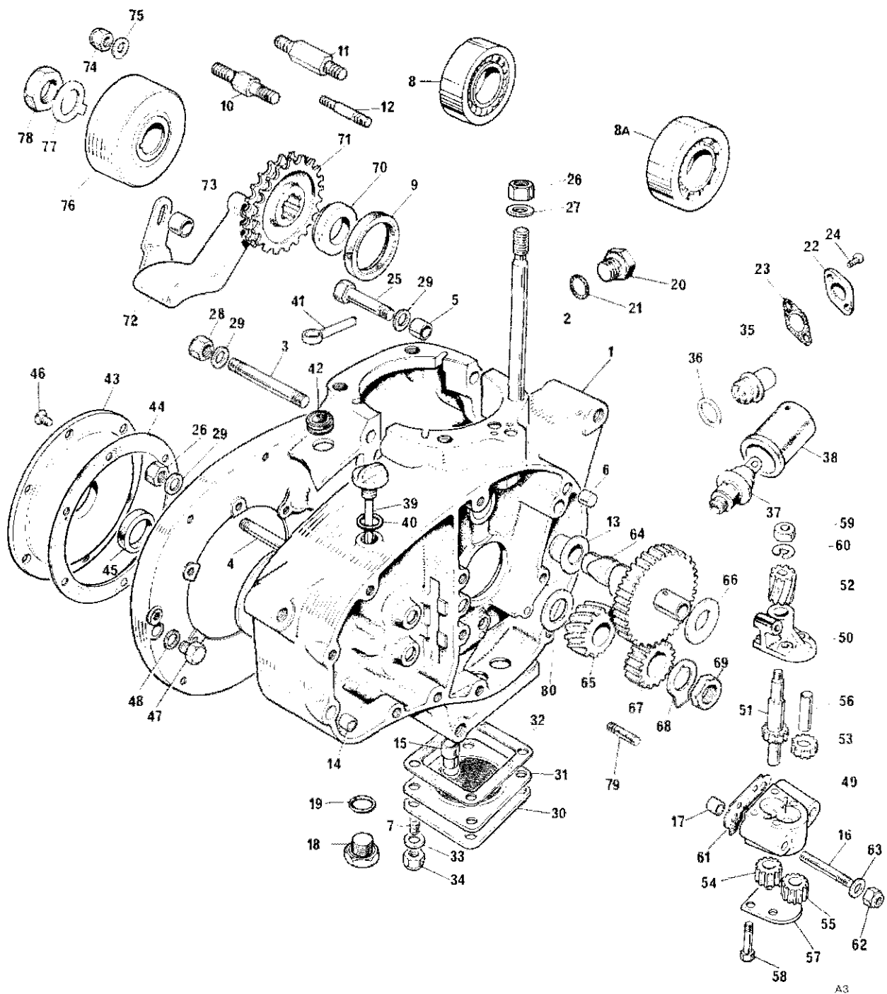
Fig. 3. CRANKCASE
