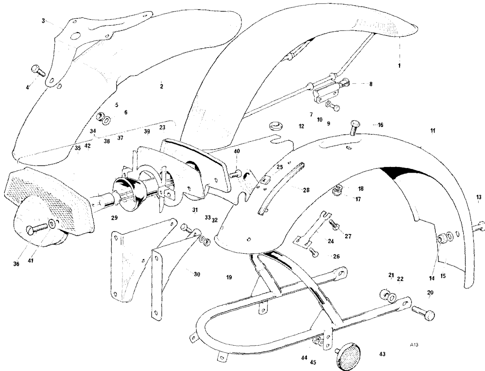
Fig. 13. FENDERS
