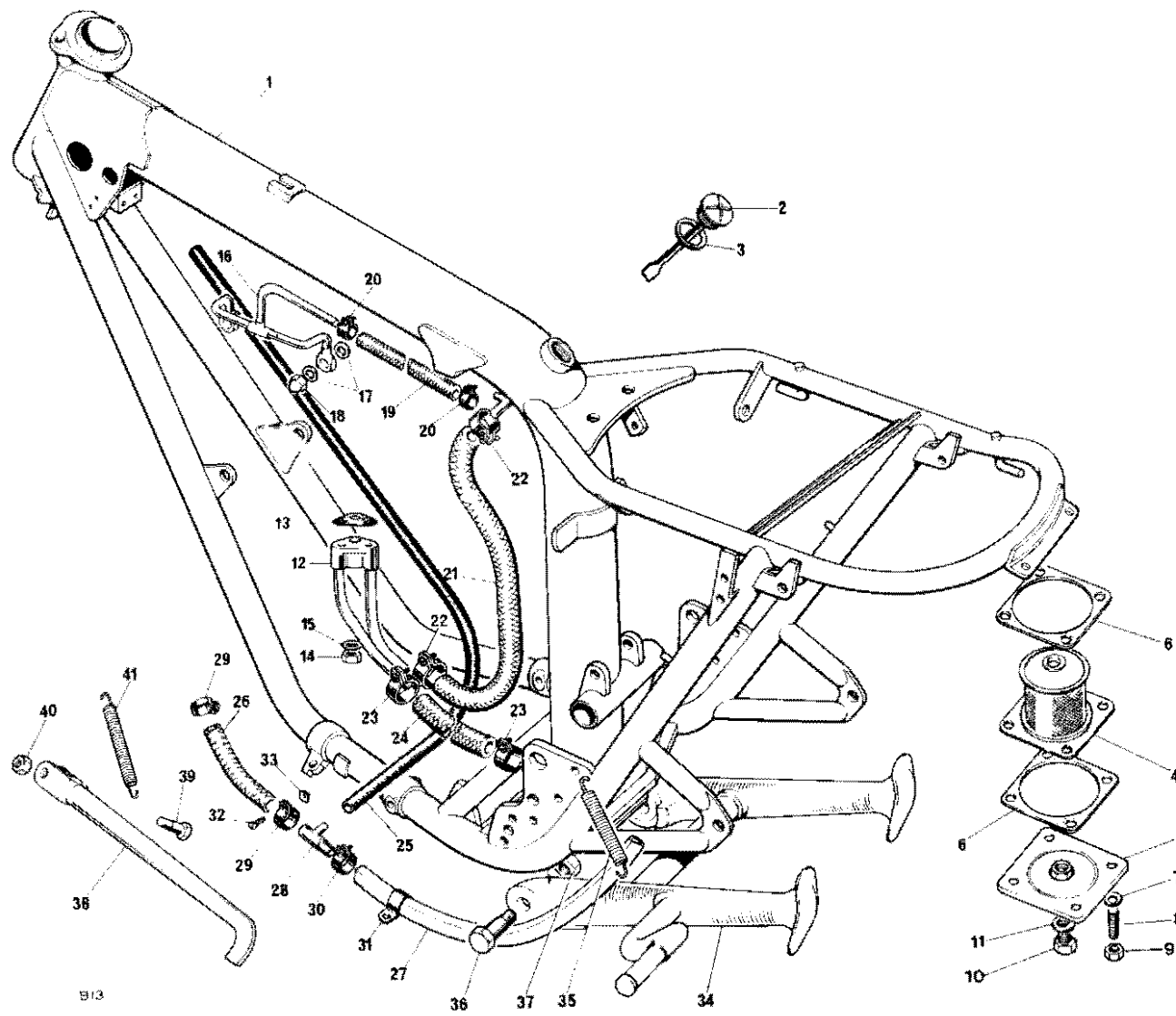
16. FRAME
