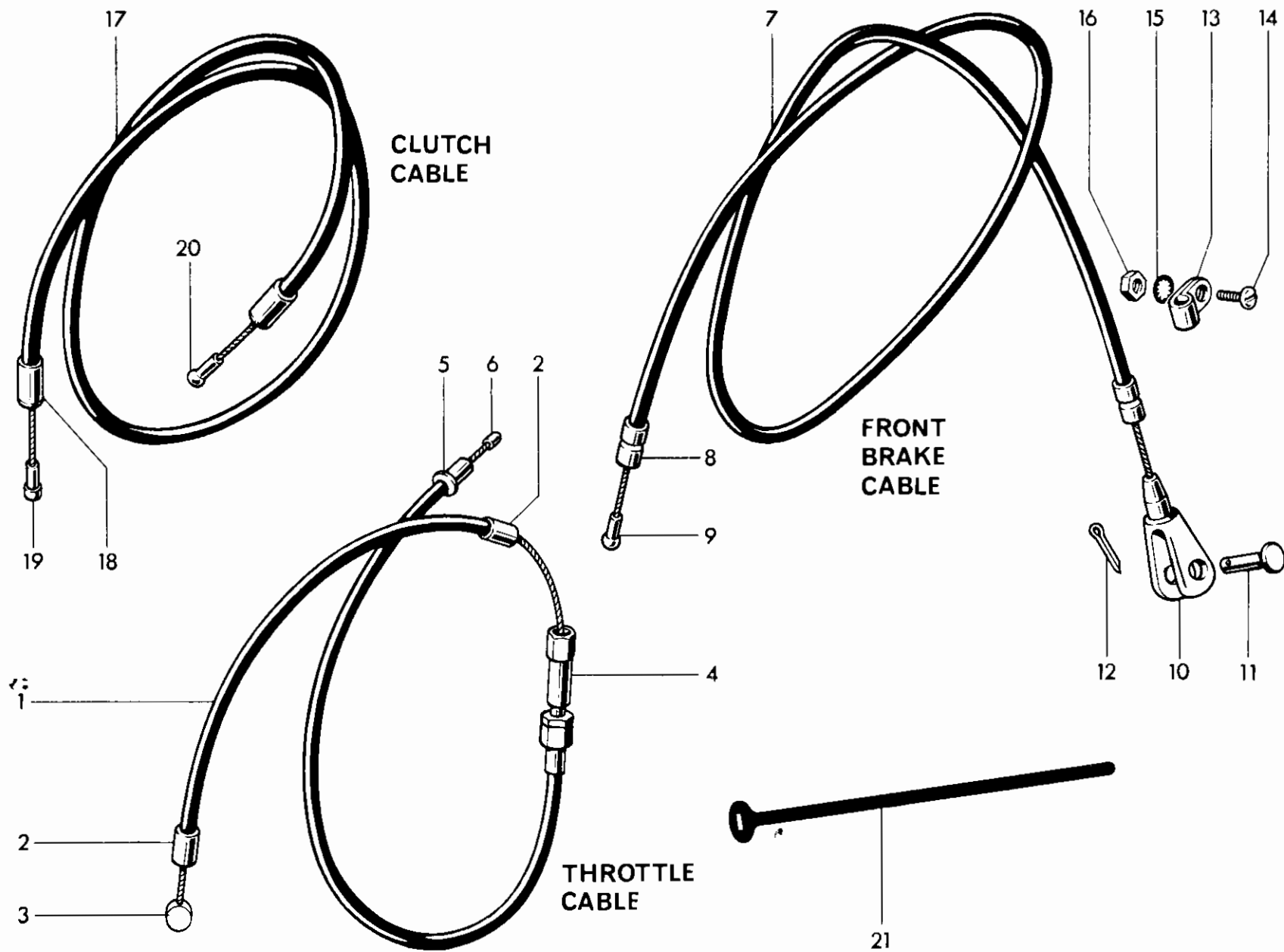
Fig. 25. CONTROL CABLES
